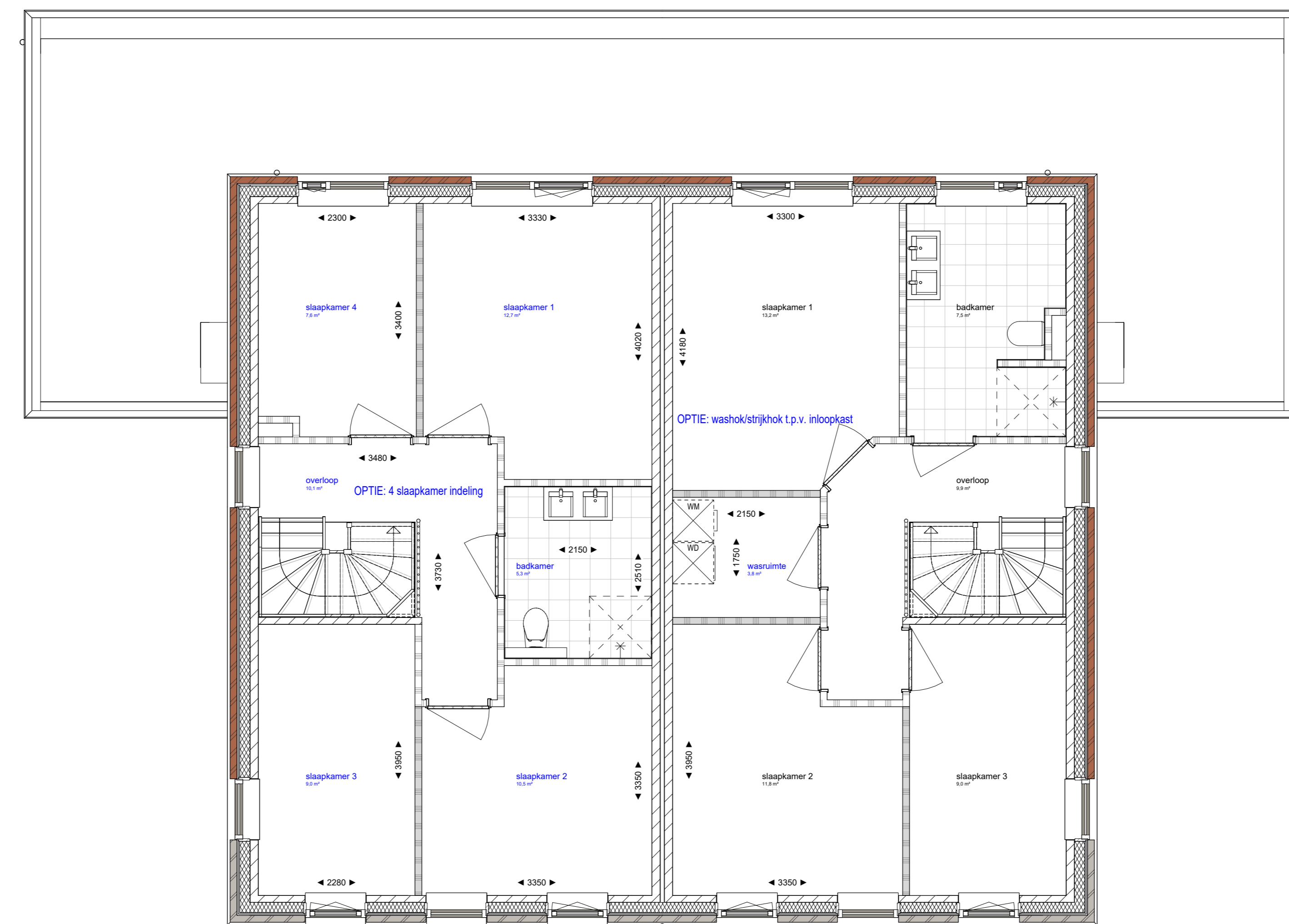
Eerste verdieping
