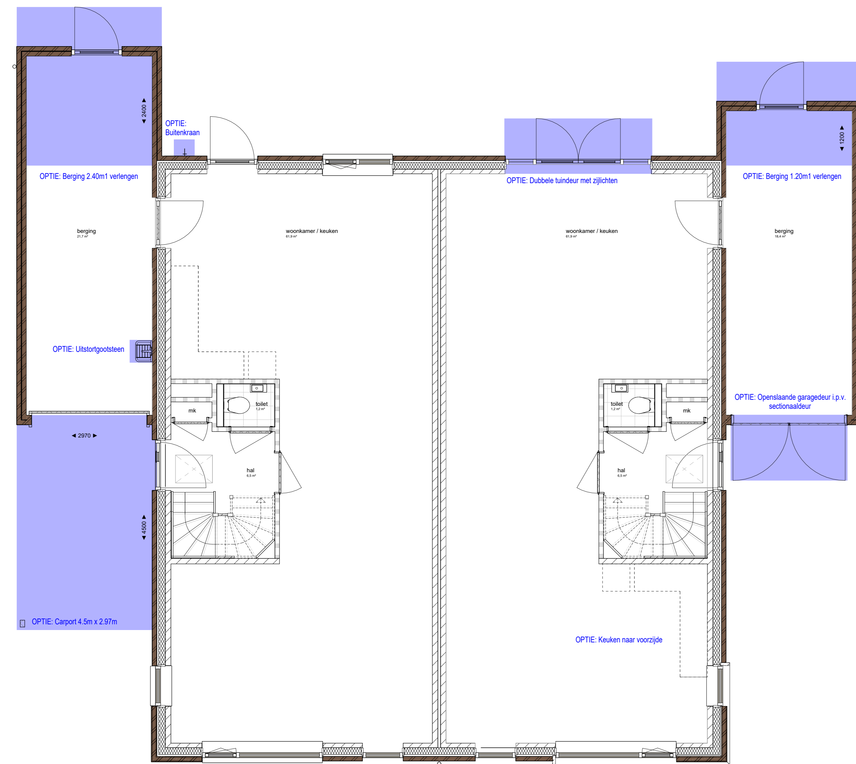
Begane grond
