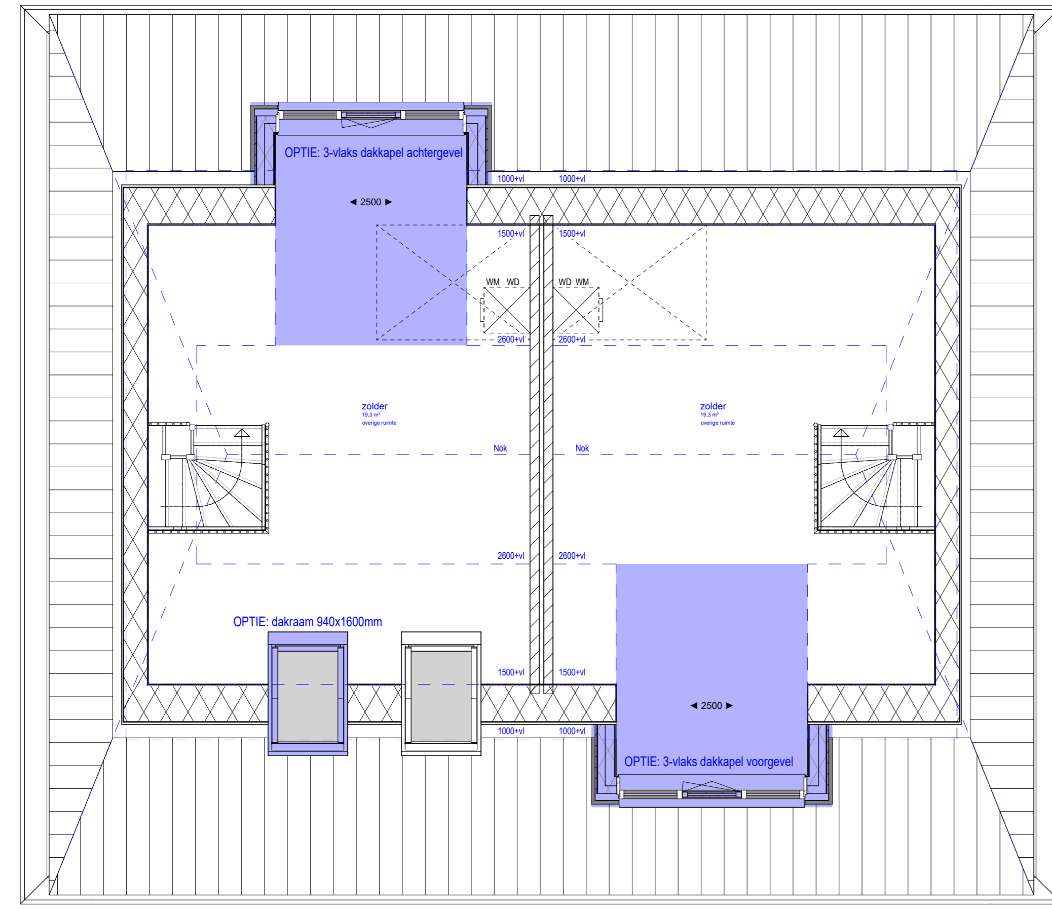
Tweede verdieping
