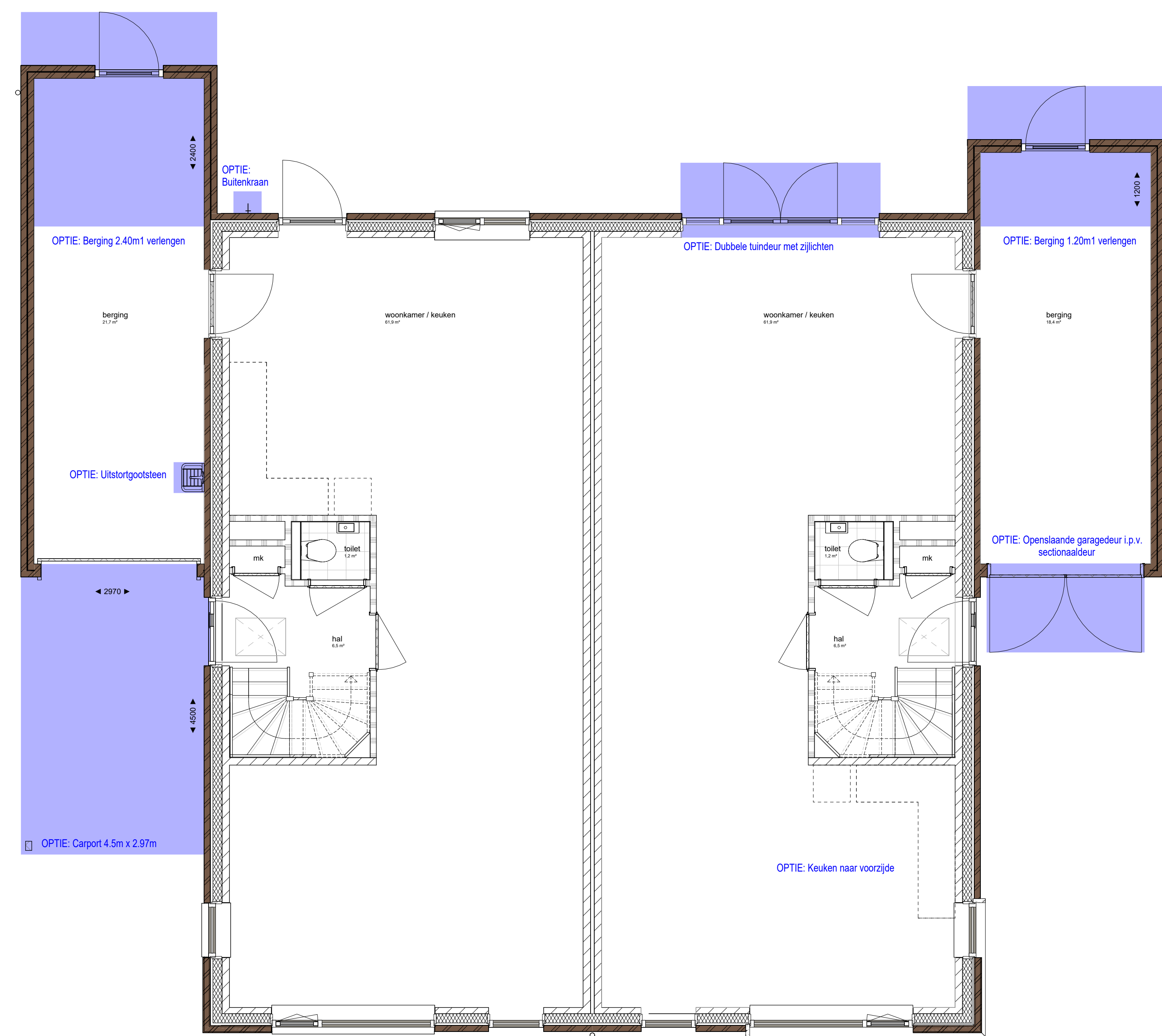
Begane grond
