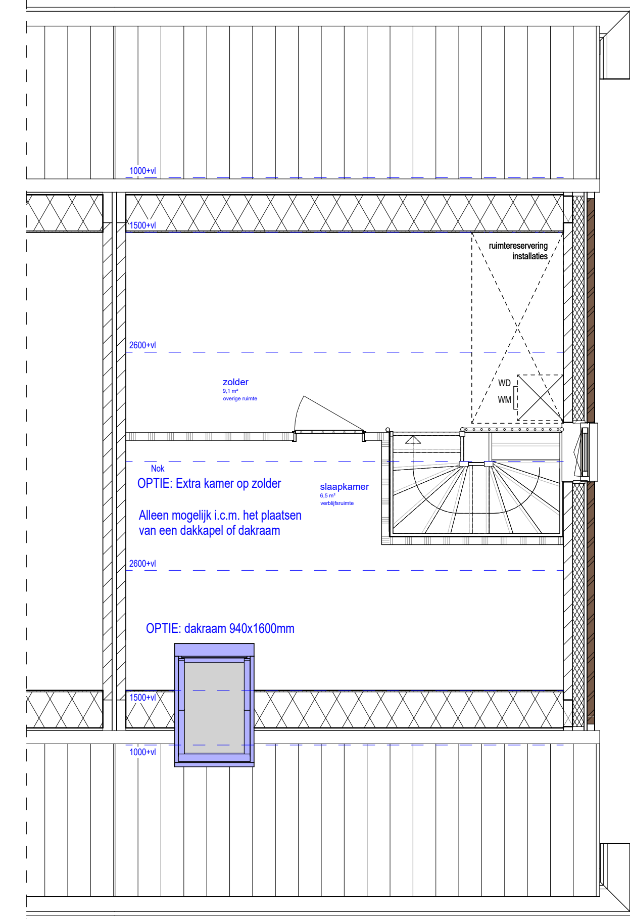
Tweede verdieping
