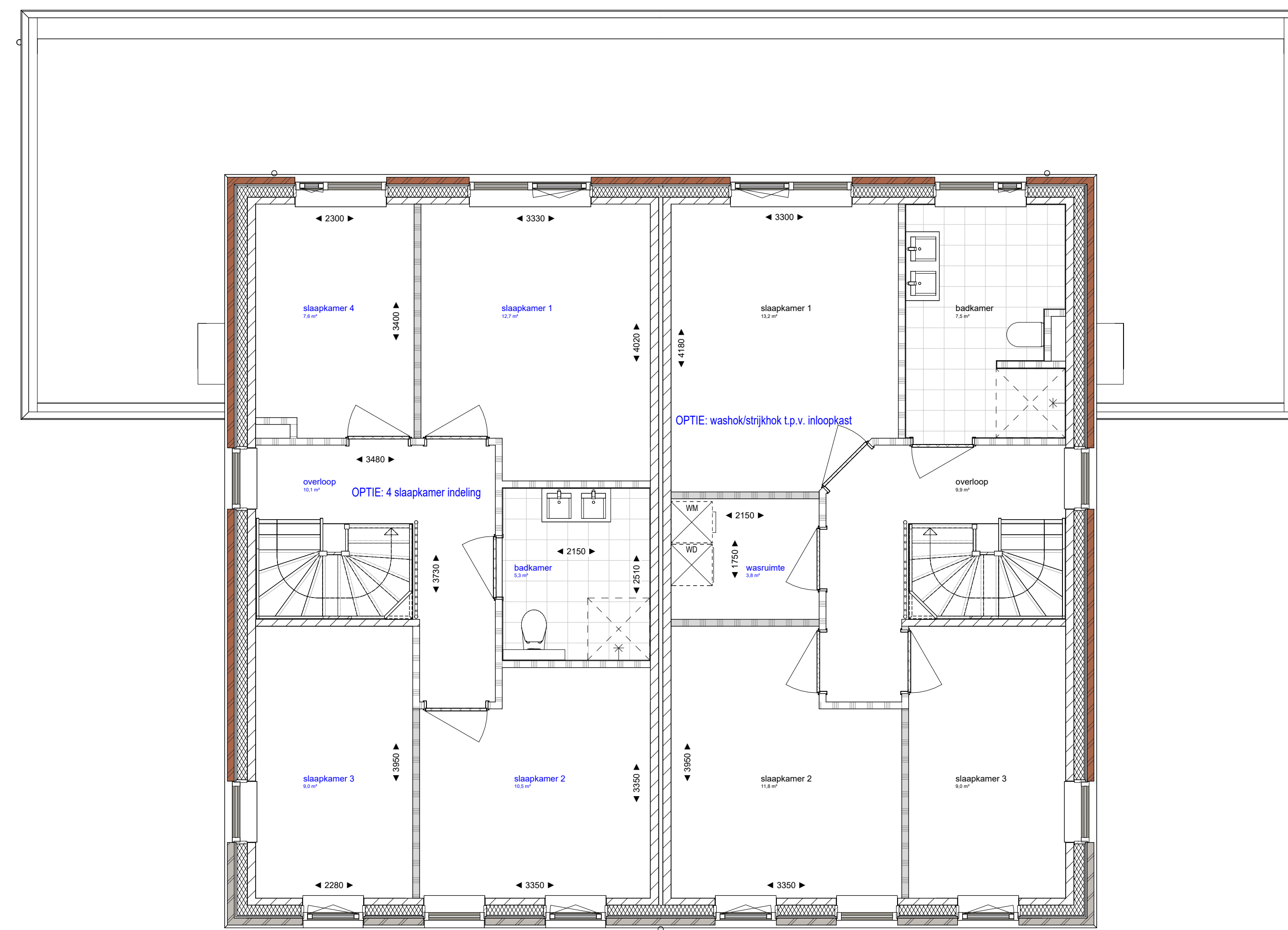
Eerste verdieping
