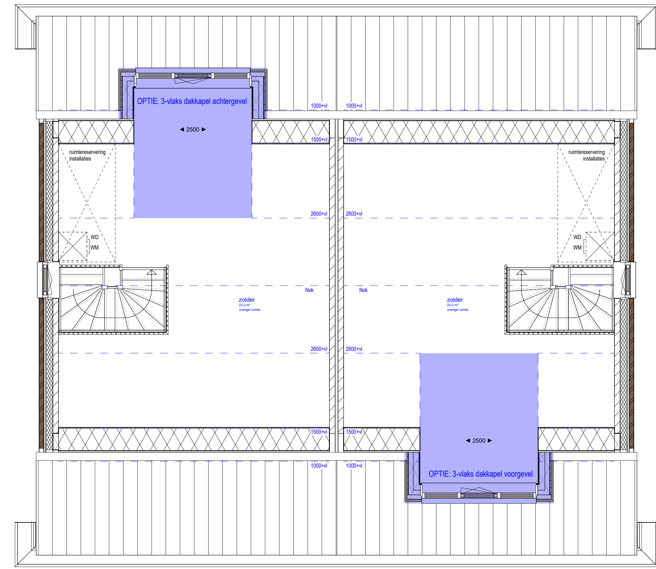
Tweede verdieping
