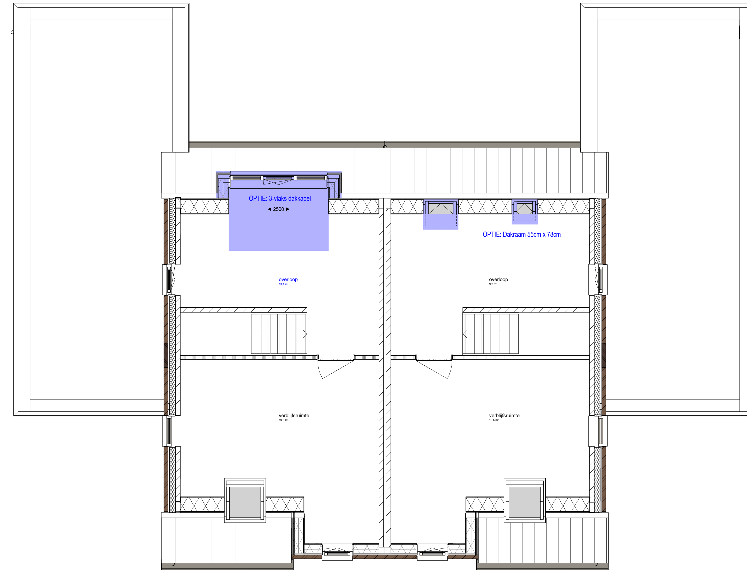
Eerste verdieping
