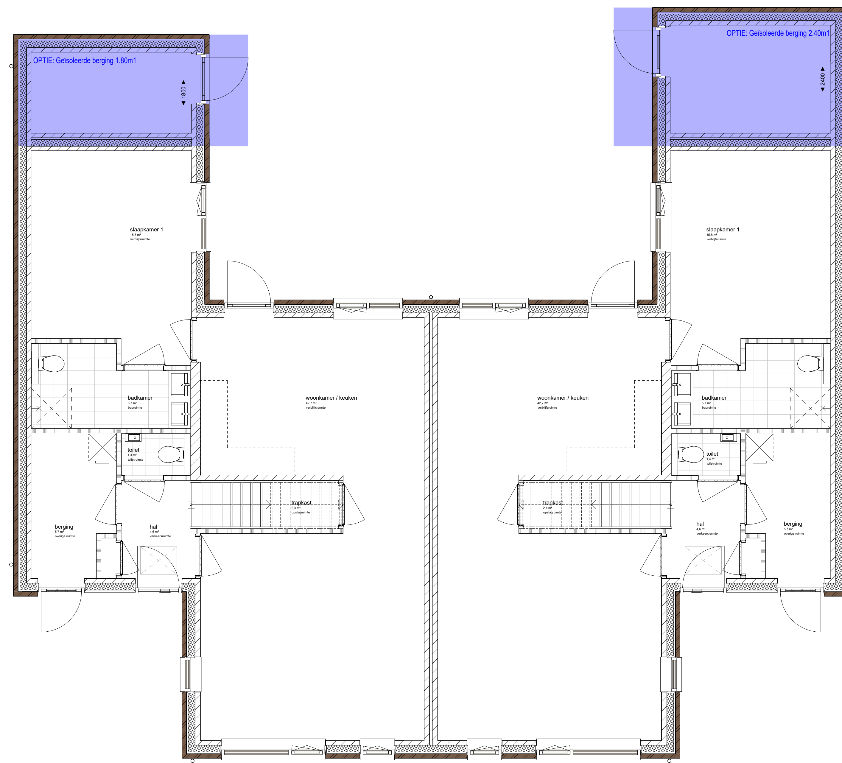
Begane grond
