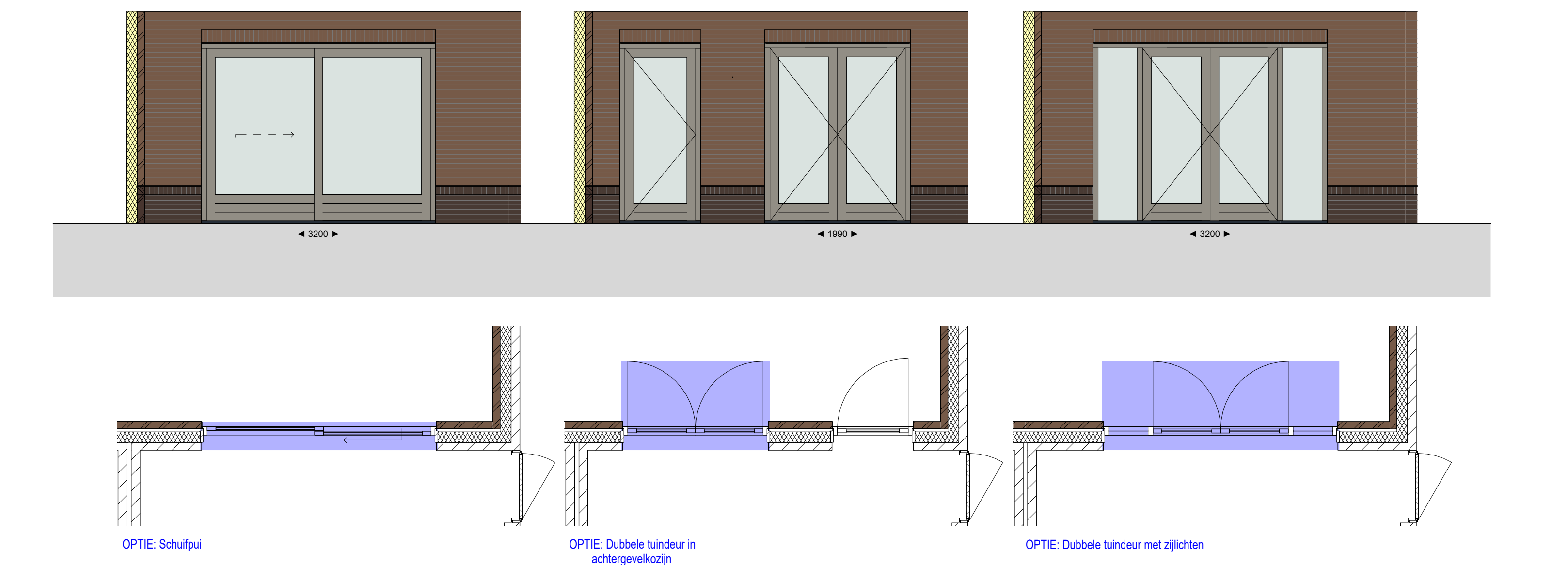
Kozijnen achtergevel
